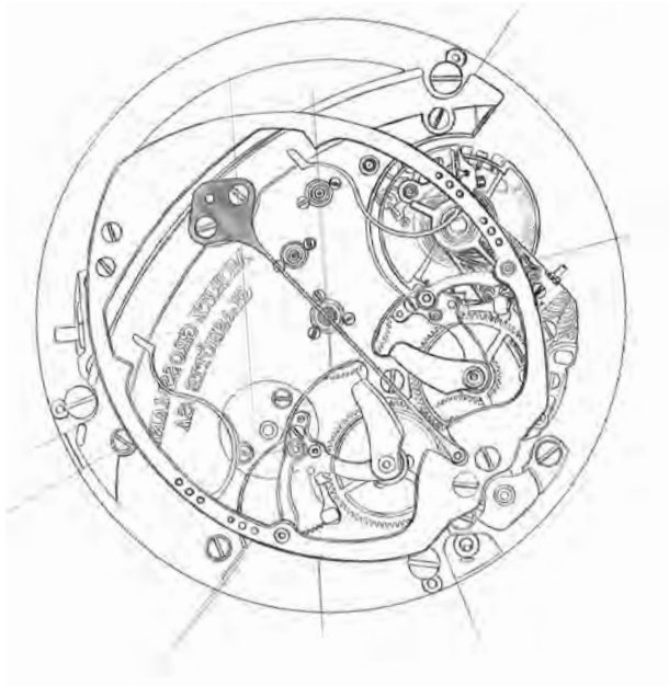
Konstruktionszeichnung Hamatic
