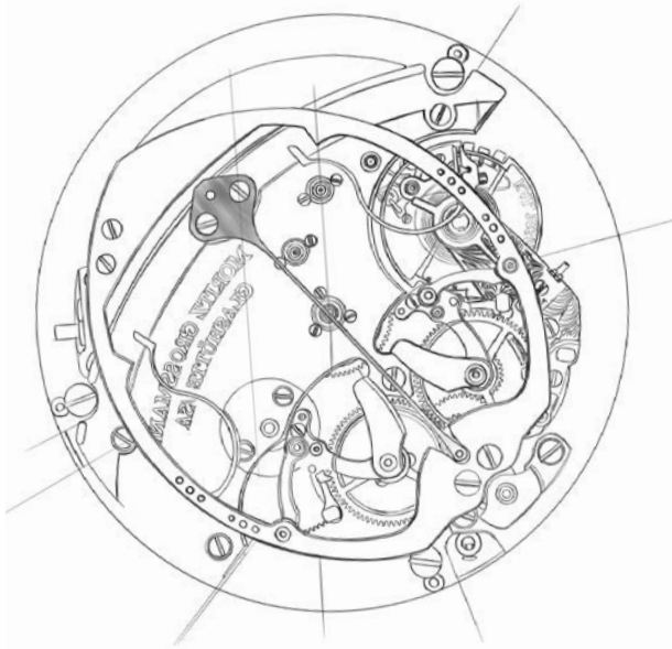
Konstruktionszeichnung Hamatic
